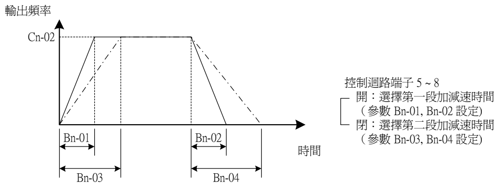
圖 11 加減速時間
