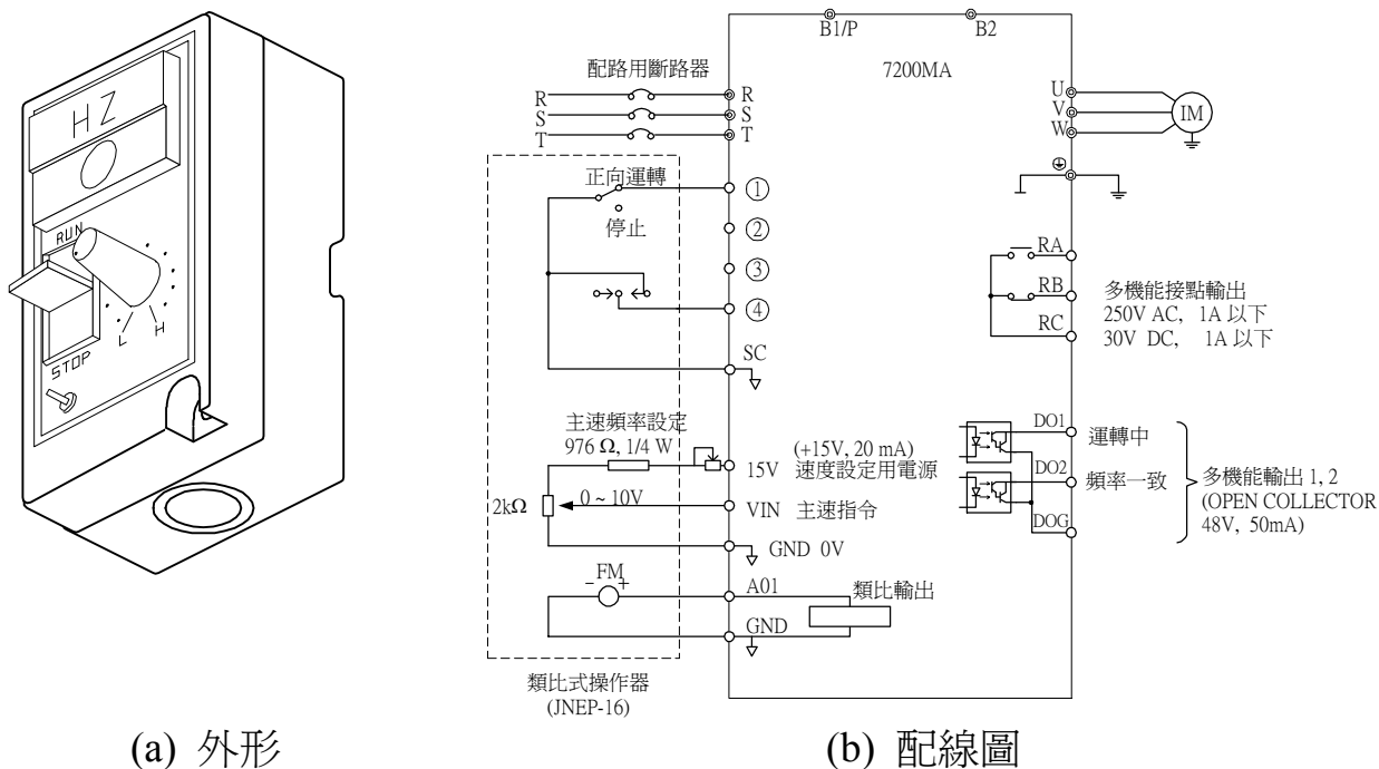
圖 9 類比操作盤
