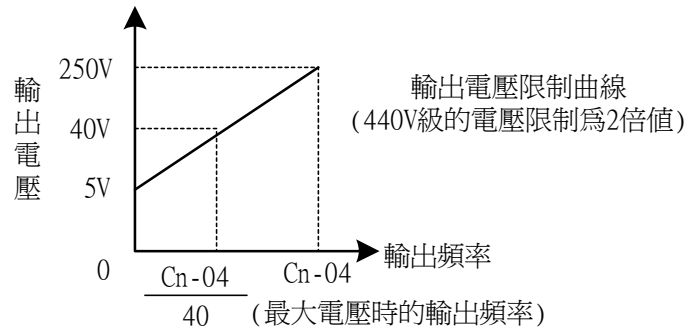
圖 34 輸出電壓限制
