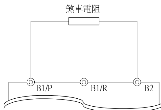
圖 7 外加煞車電阻接線圖
