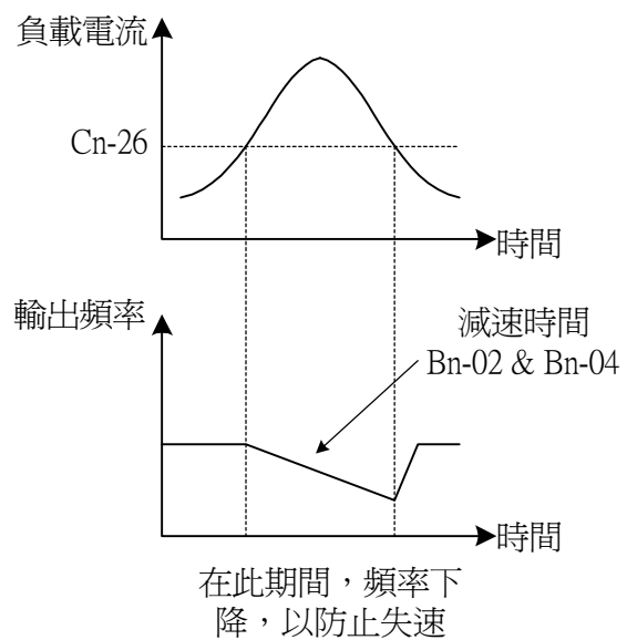
圖 25 運轉中失速防止機能
