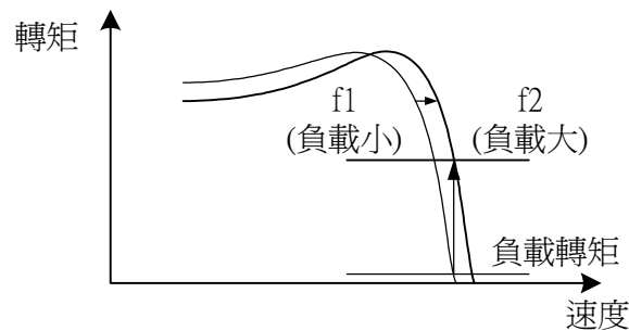
圖 19 滑差補正控制
