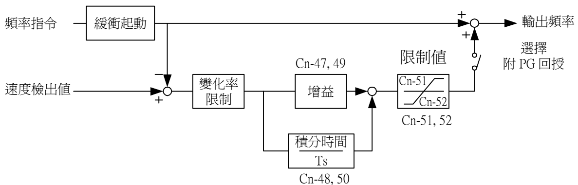
圖 44 PG 速度控制方塊圖
