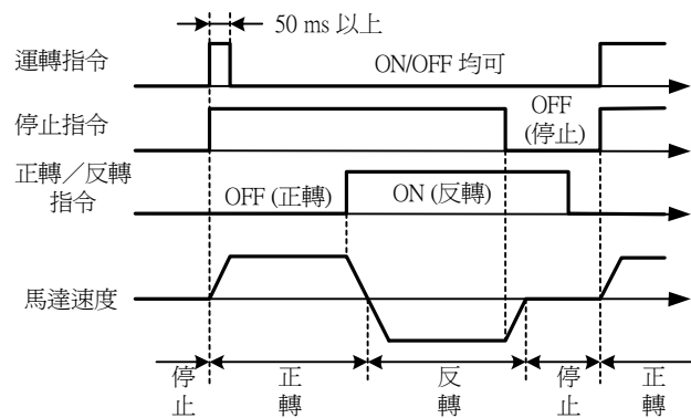
圖 39 3 線式運轉順序圖
