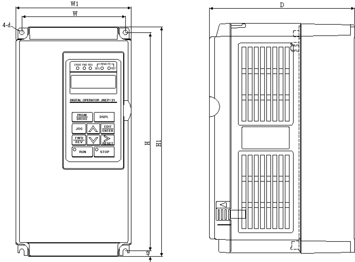
圖 6 變頻器外形尺寸圖
